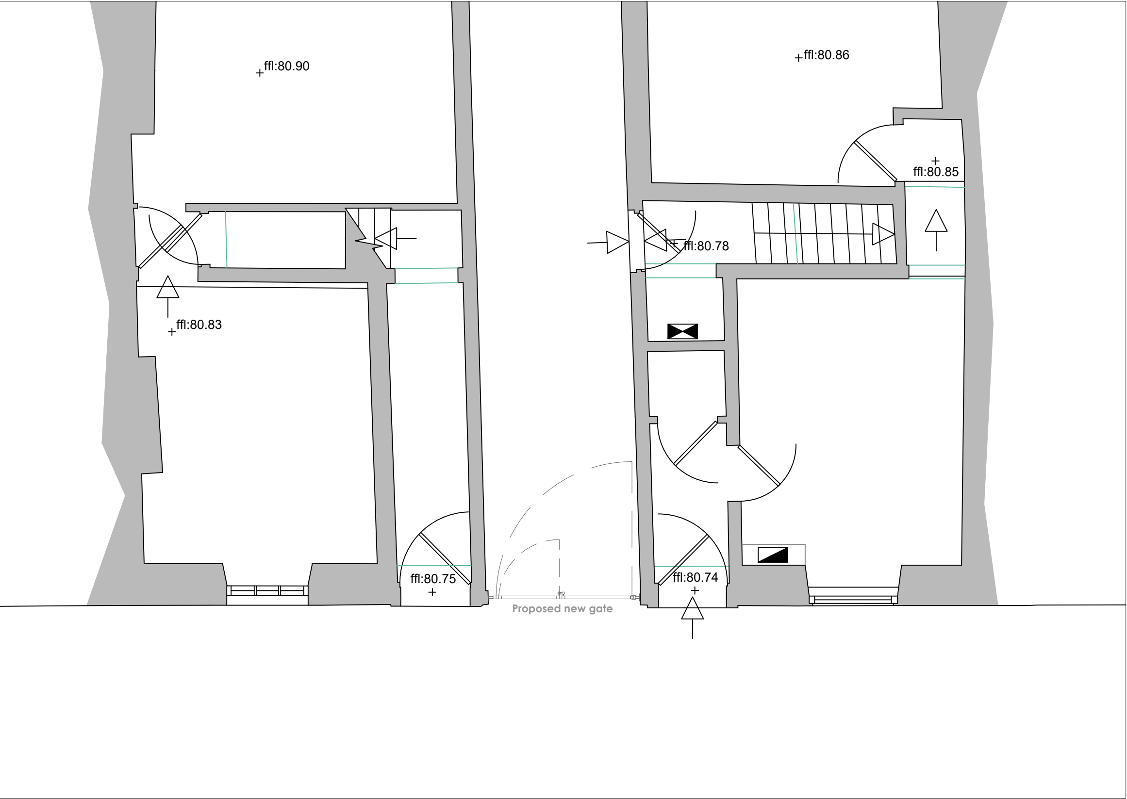
Plan 1:50
