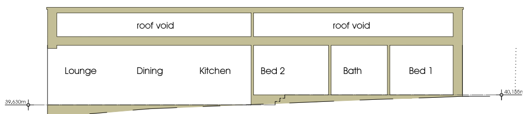
Longitudinal Section scale 1:100
