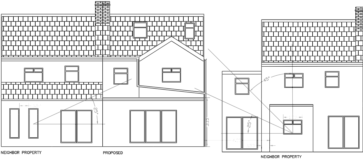
ELEVATION 1:100
