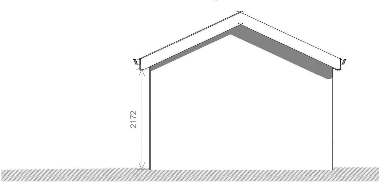
3 Elevation 3 1 : 50
