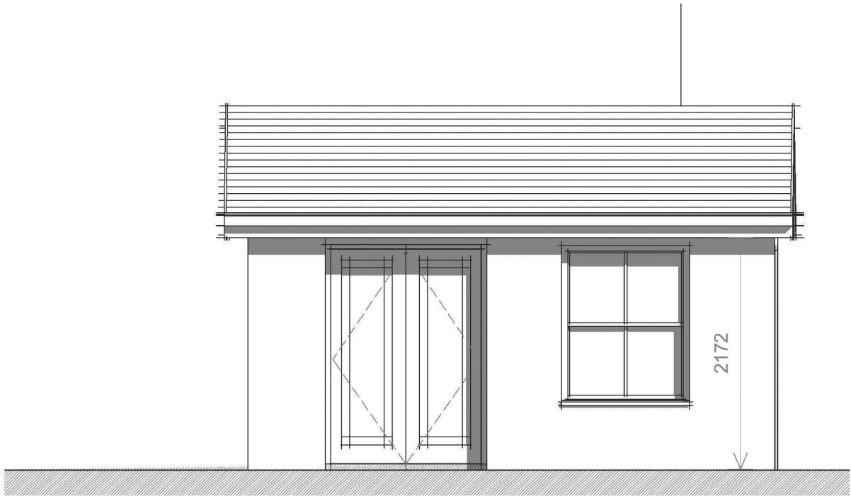
1 Elevation 1 1 : 50
