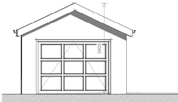
② Elevation 2 1 : 50
