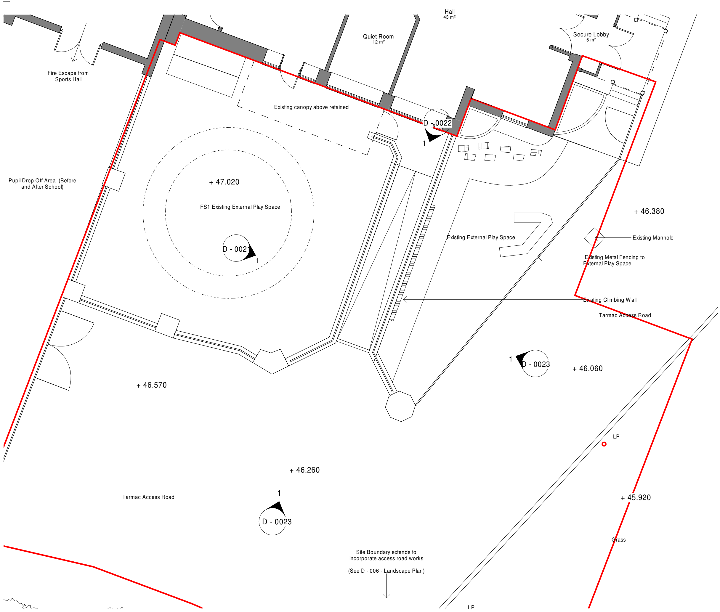
1 Existing Site Plan 1 : 100
