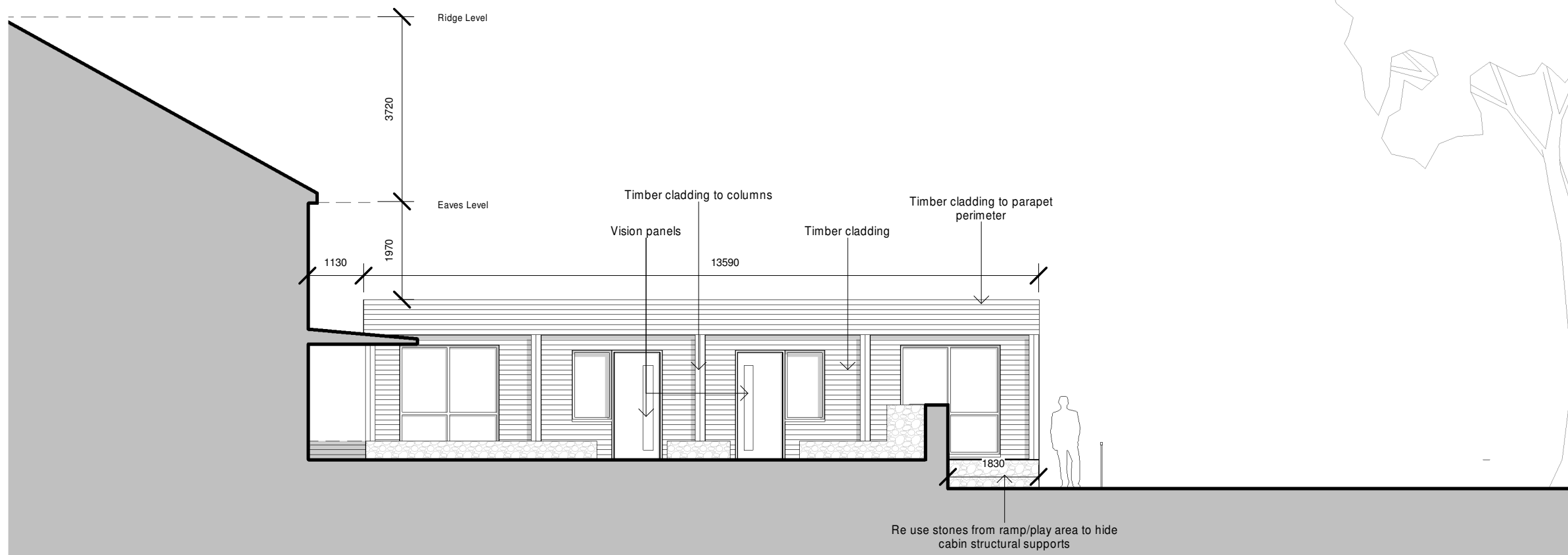
1 NW Elevation 1 : 100
