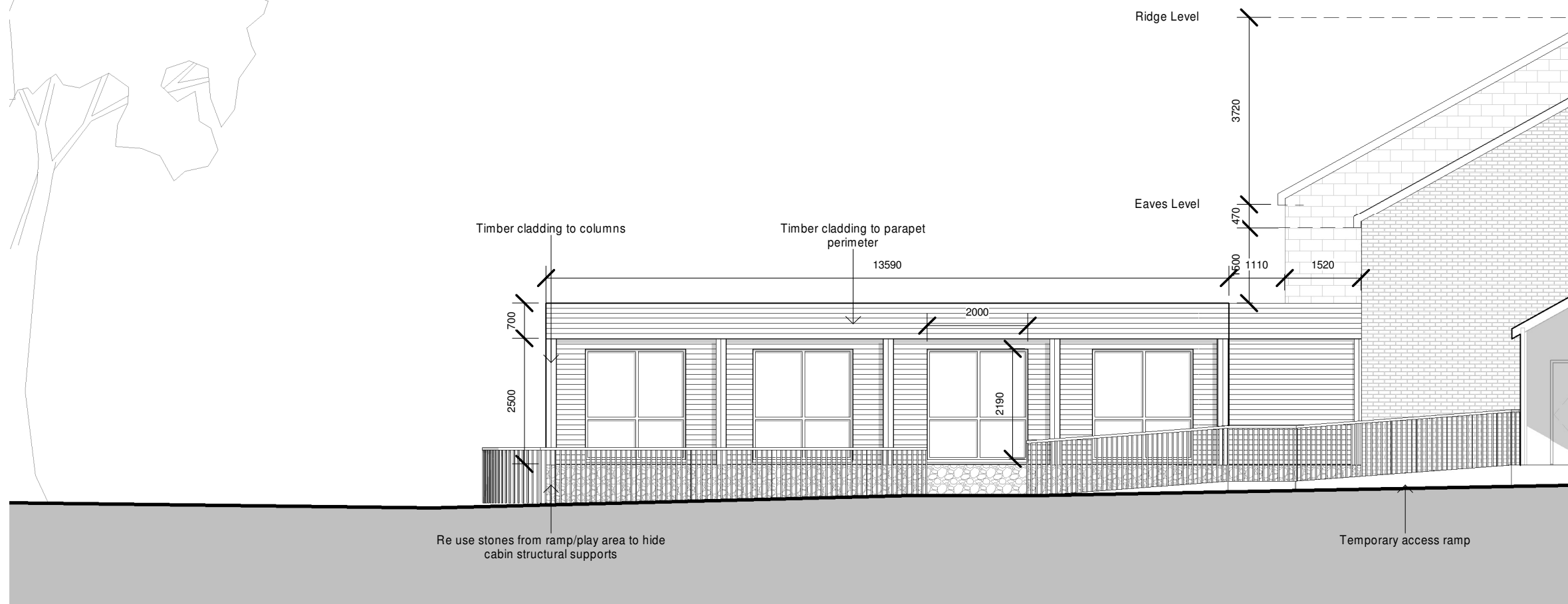
1 SE Elevation 1 : 100
