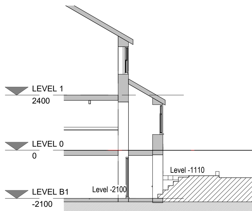
2 Existing Section 1 : 100
