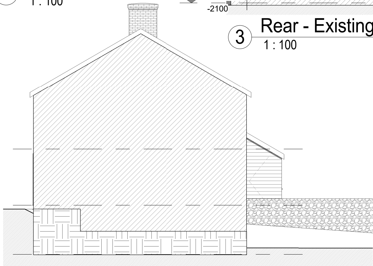
4 Right Side - Existing 1 : 100
