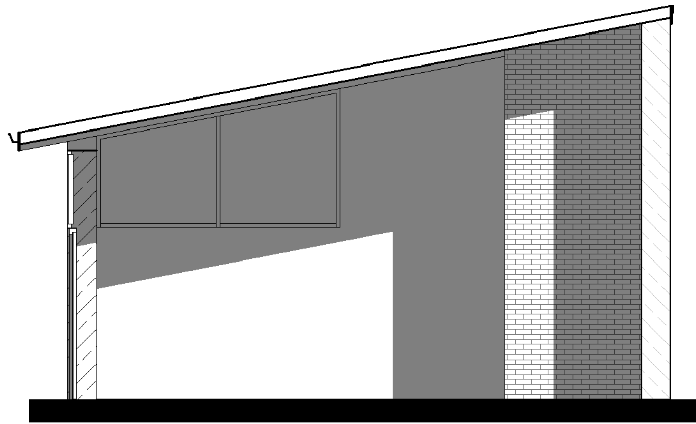
6 Section 1 1 : 50
