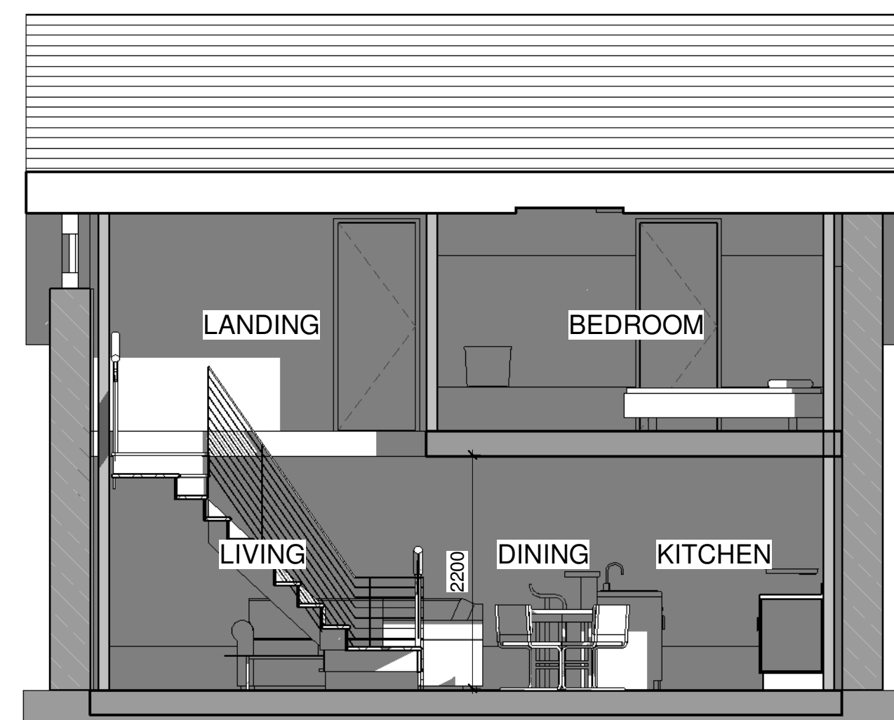
6 Section 1 1 : 50
