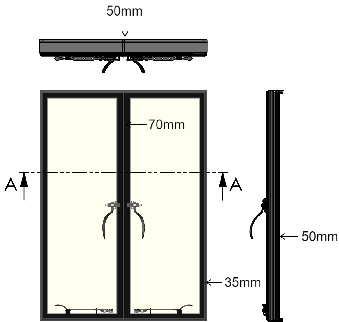
SCALE 1 : 10
