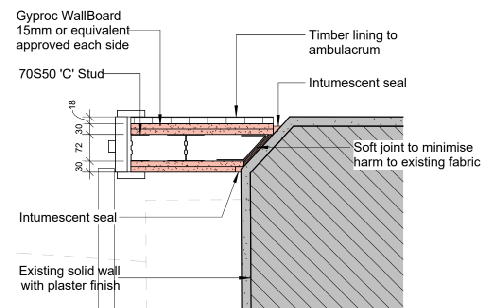
3 | Wall Jamb Detail
