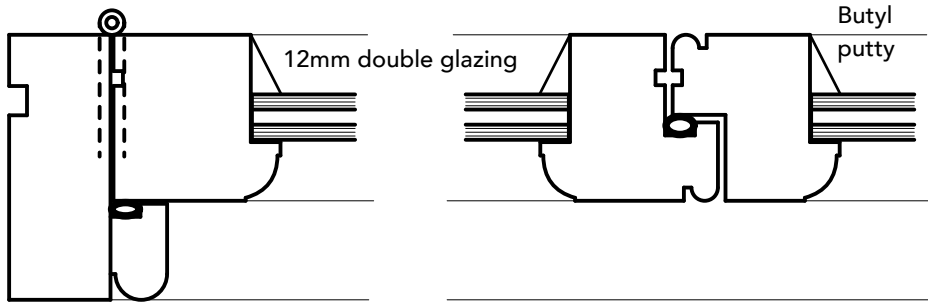
Horizontal Section 1:2
