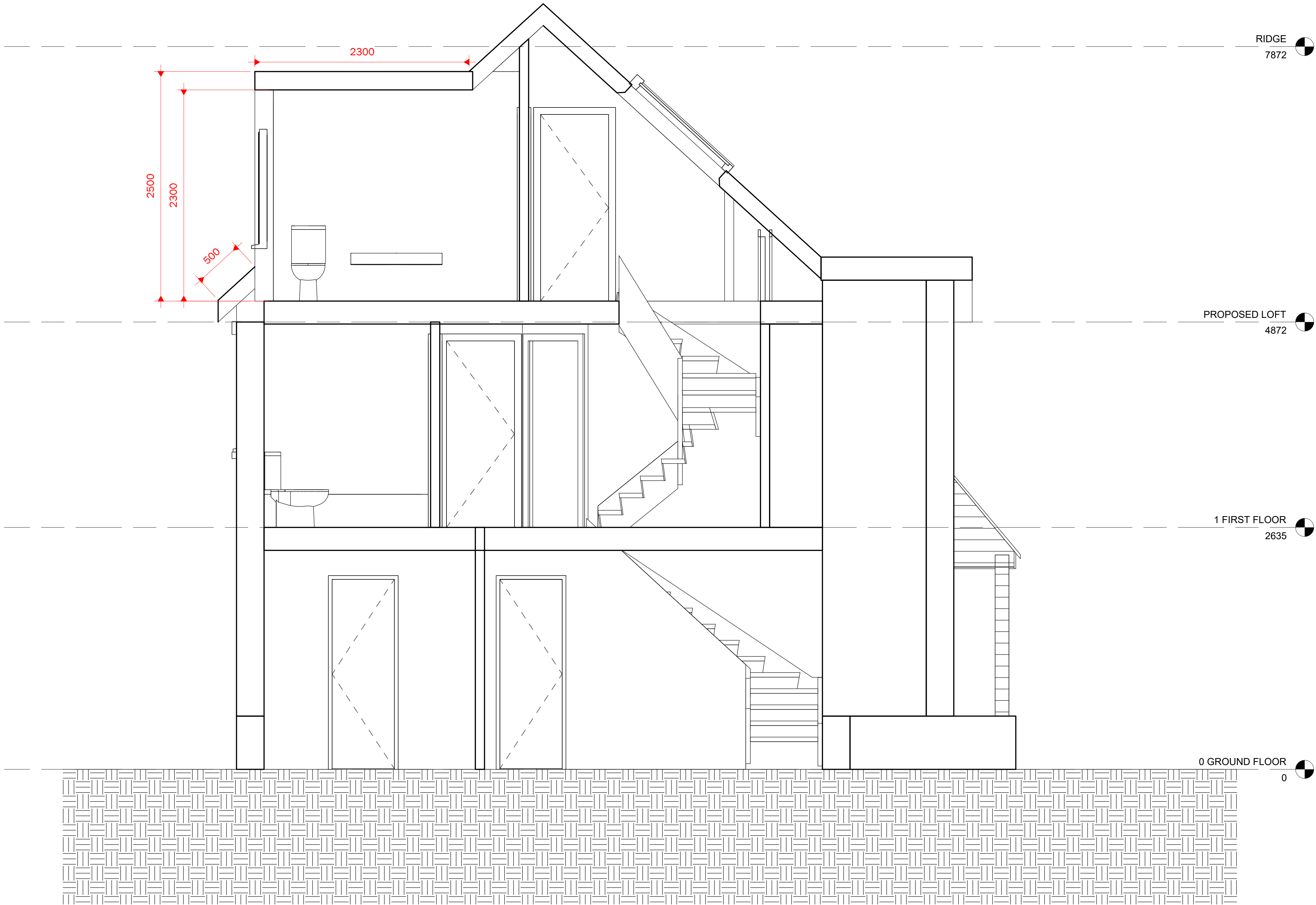
1 Section 1 1 : 25
