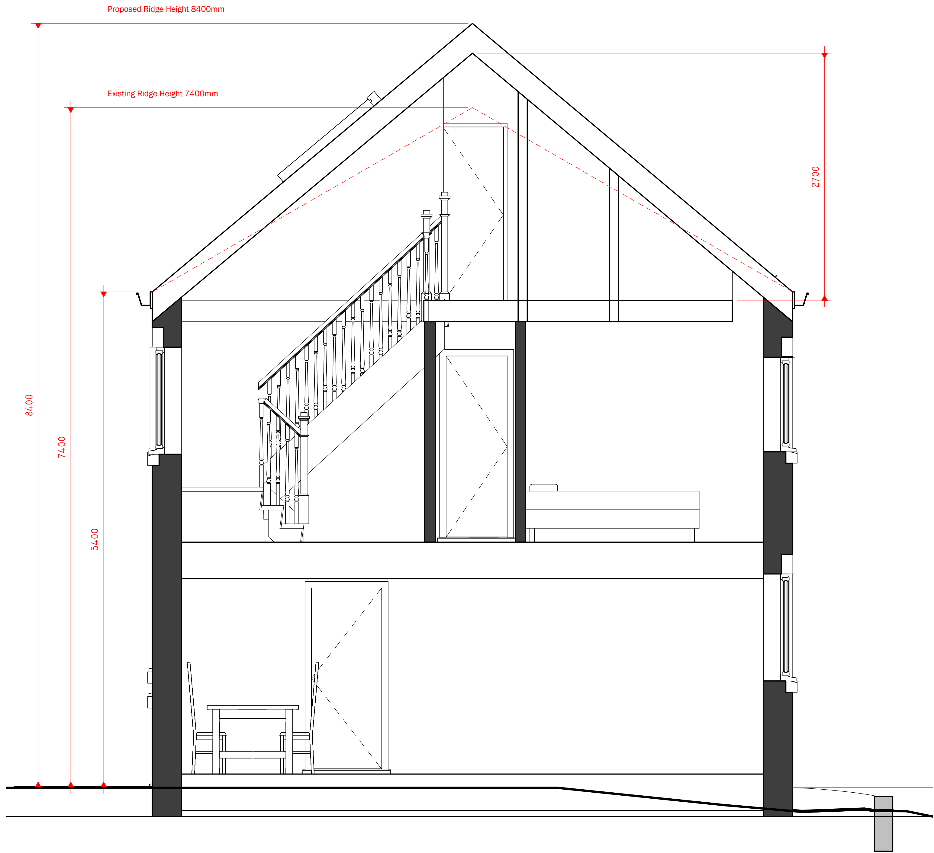
1 Section 1 1 : 25
