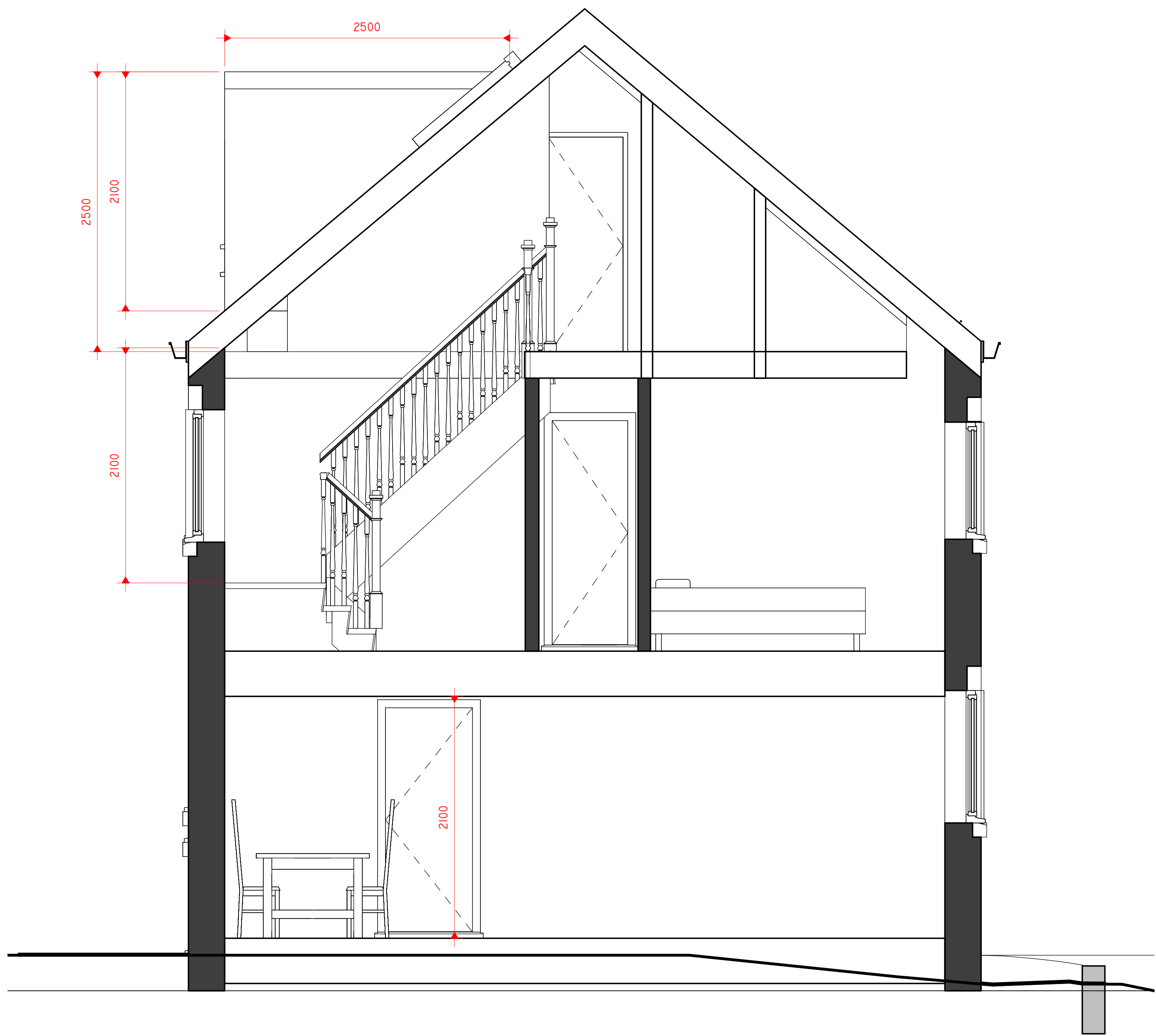
1 Section 1 1 : 25
