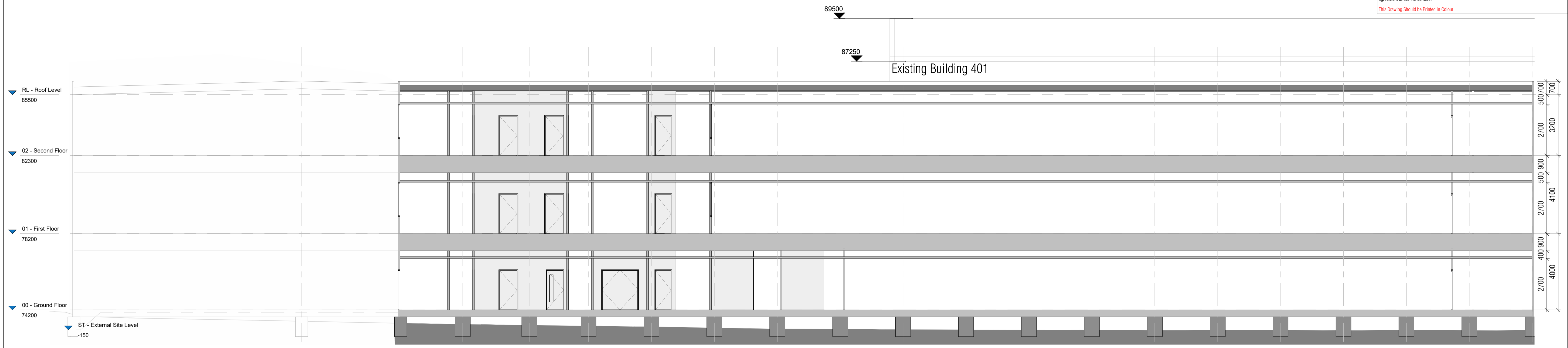
A-A Section A-A 1:100
