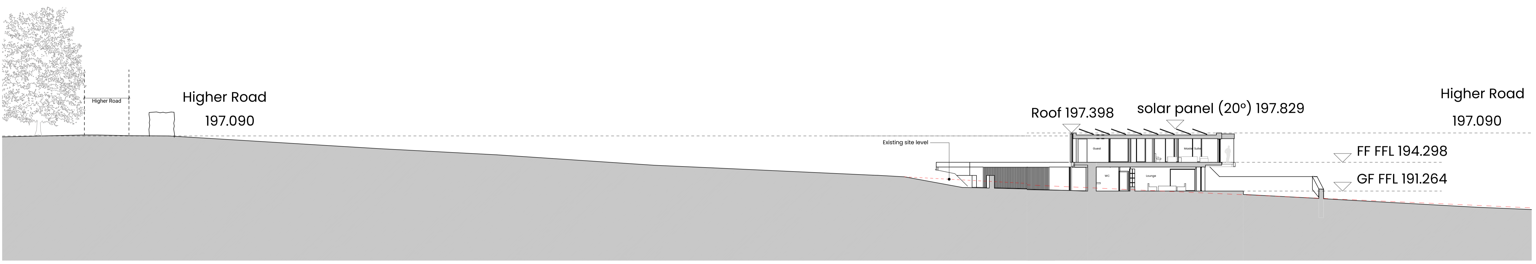
Section D-D 1:200
