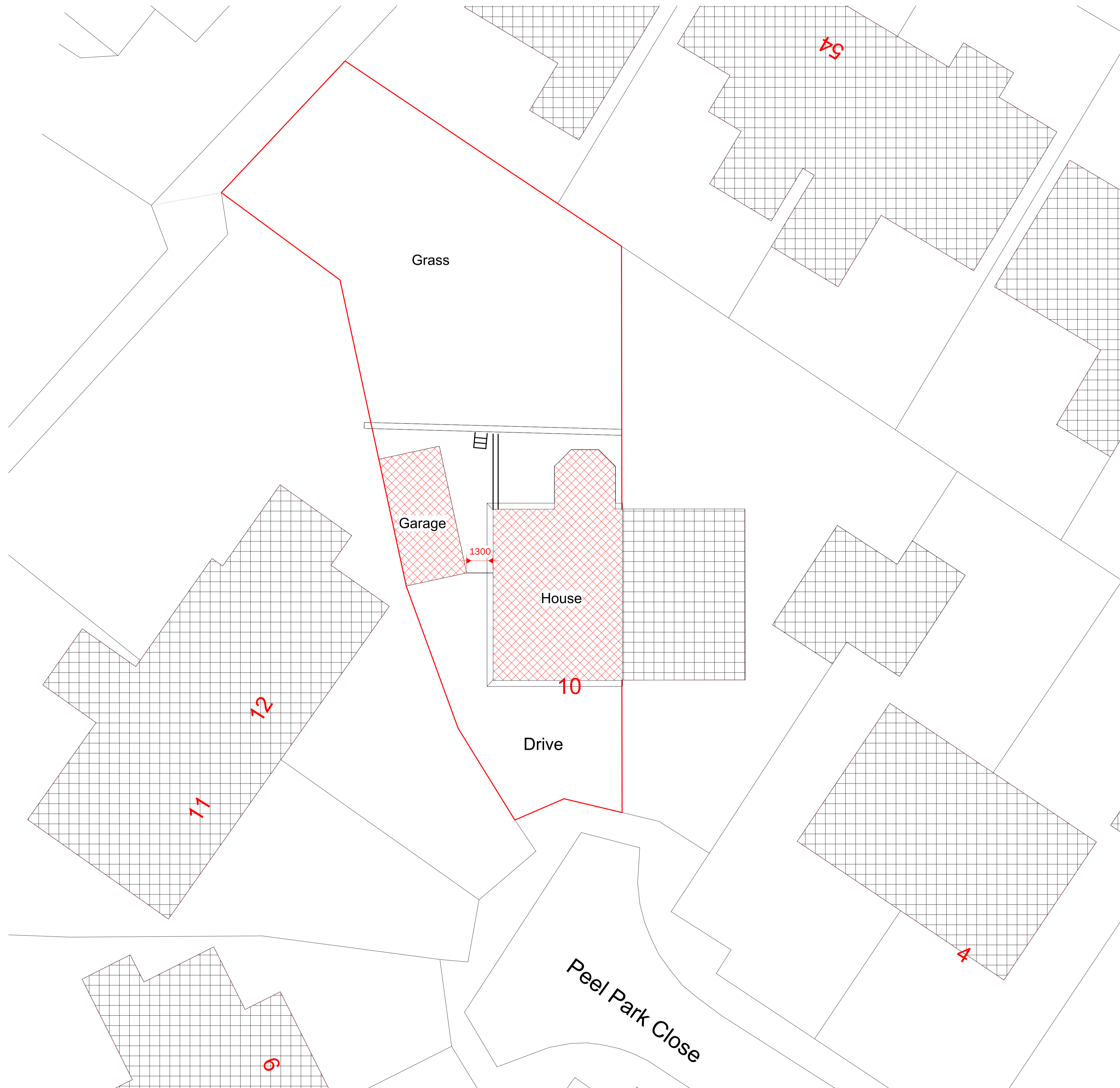
1 EXISTING SITE PLAN 1 : 100
