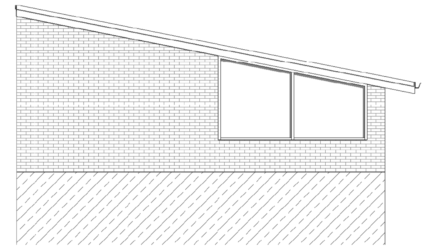
5 Side Elevation 2 1:50
