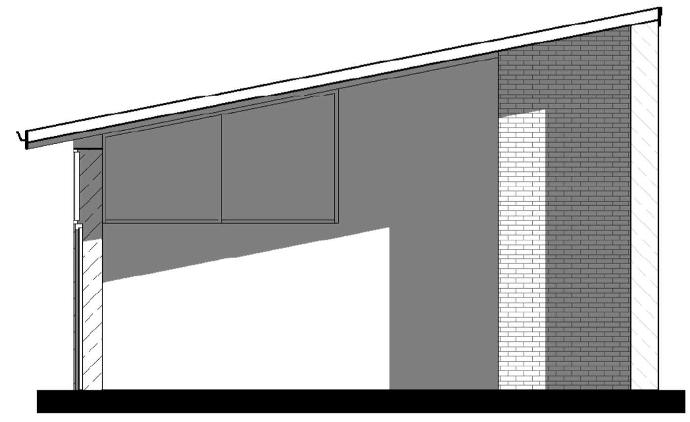
6 Section 1 1:50
