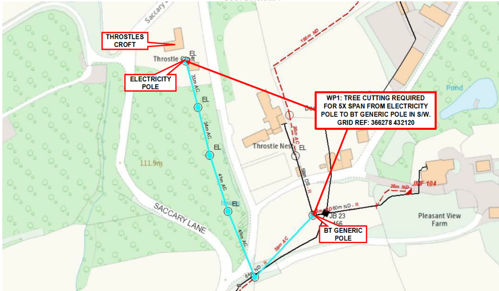
-DUCT DIAGRAM-1-
