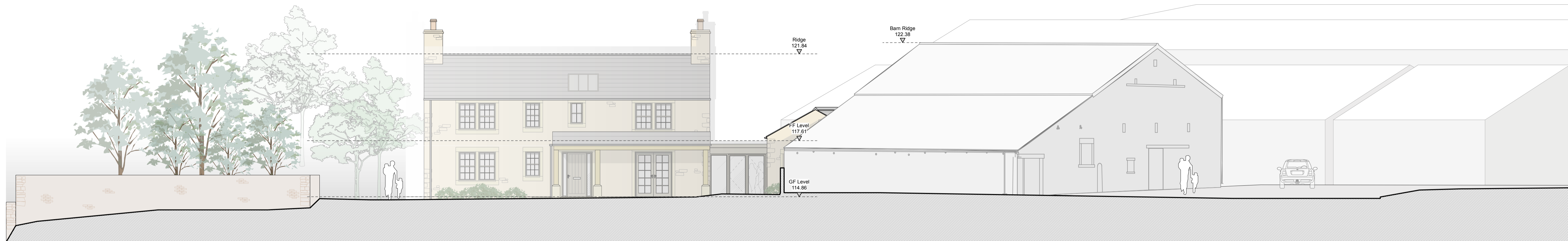
Site Section A,A 1:100
