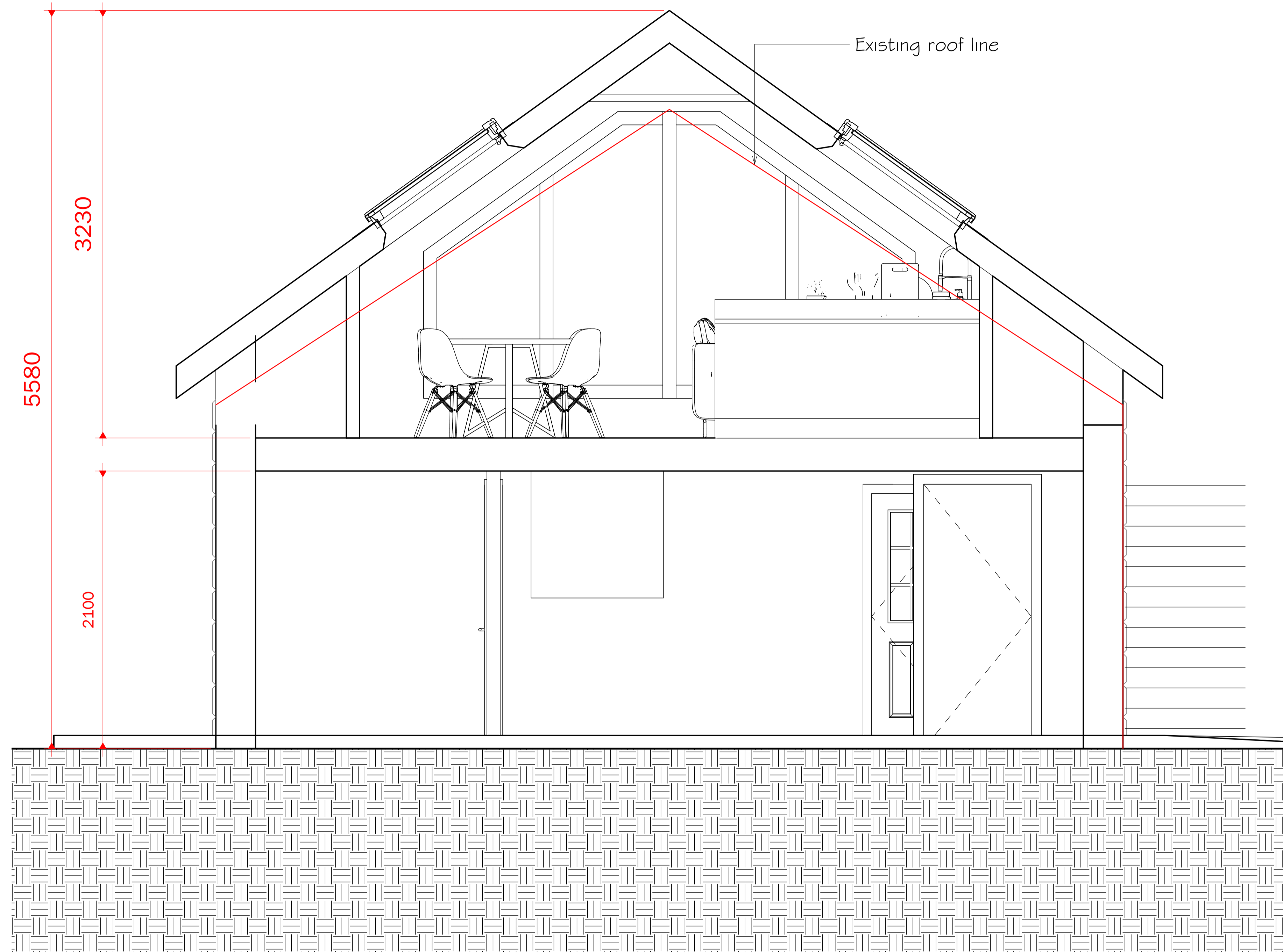
1 Section 1 1 : 20
