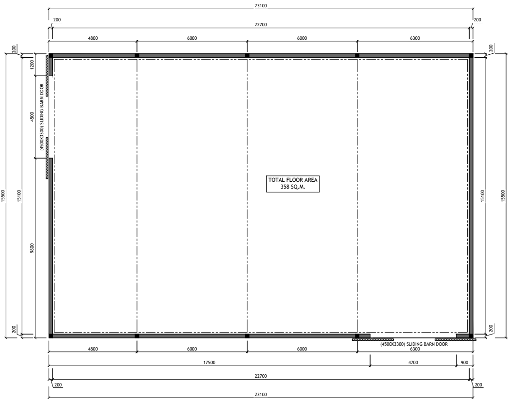
1 FLOOR PLAN SCALE: 1:200 @ A3
