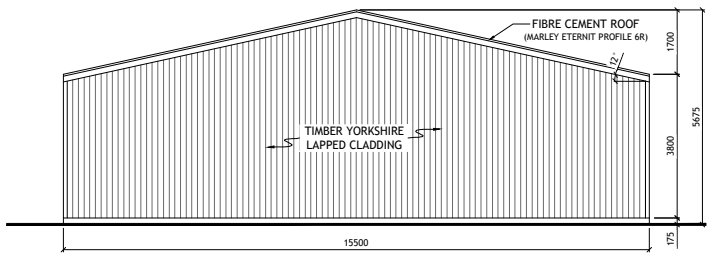
2 SOUTH ELEVATION SCALE: 1:200 @ A3
