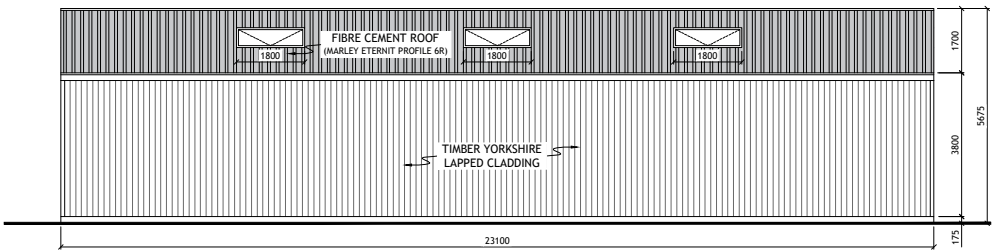
5 EAST ELEVATION SCALE: 1:200 @ A3
