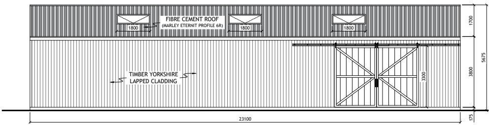
4 WEST ELEVATION SCALE: 1:200 @ A3
