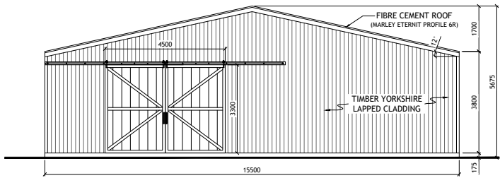
3 NORTH ELEVATION SCALE: 1:200 @ A3
