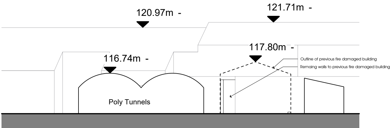
3 Existing Street Scene Scale: 1:200
